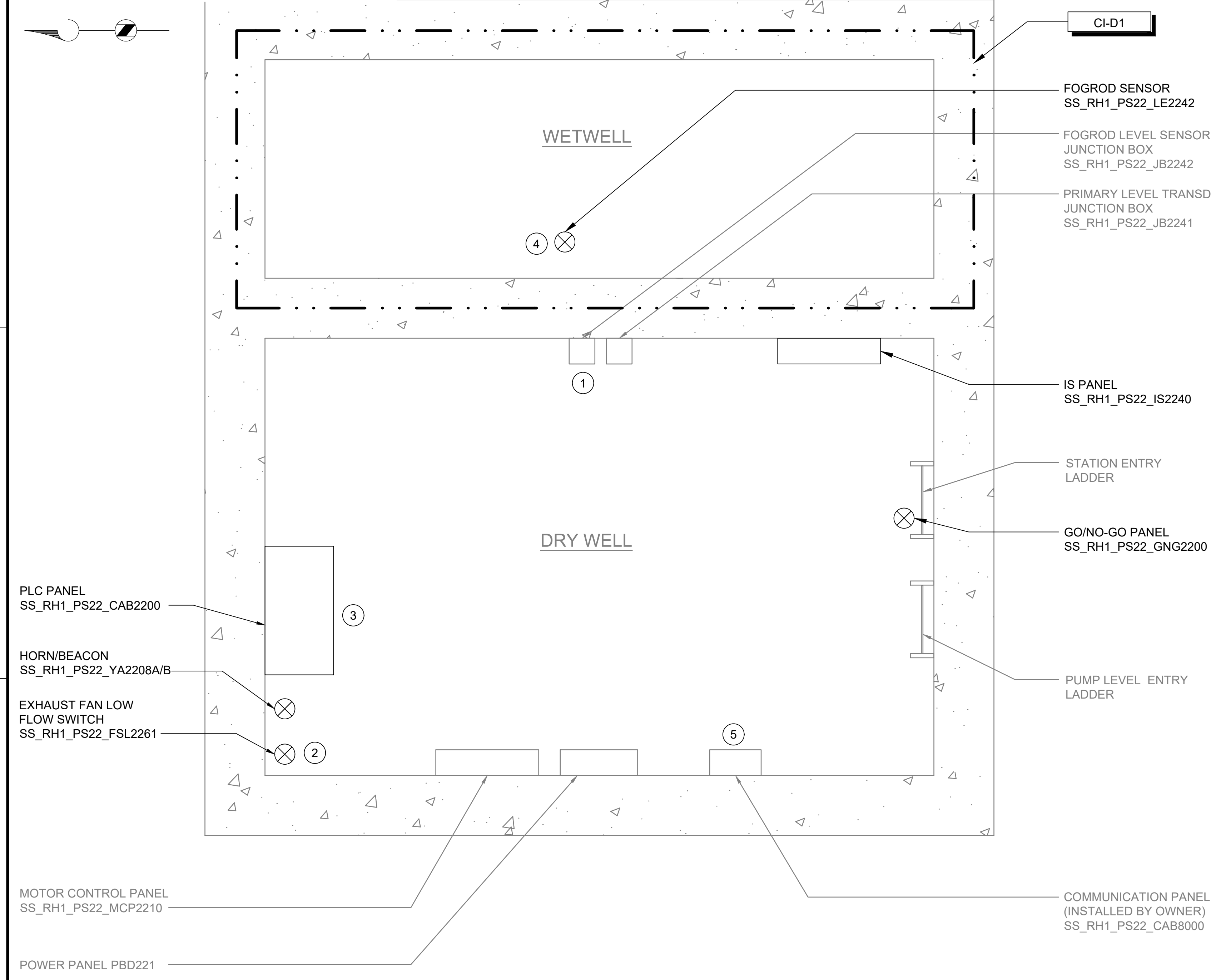
PLAN SCALE: 3/4" = 1'-0"
